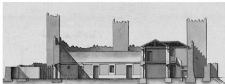
Sección de la fortaleza en el proyecto de cuartel de 1740.
